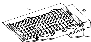
VFR Schwerlastkeil Einteilig
